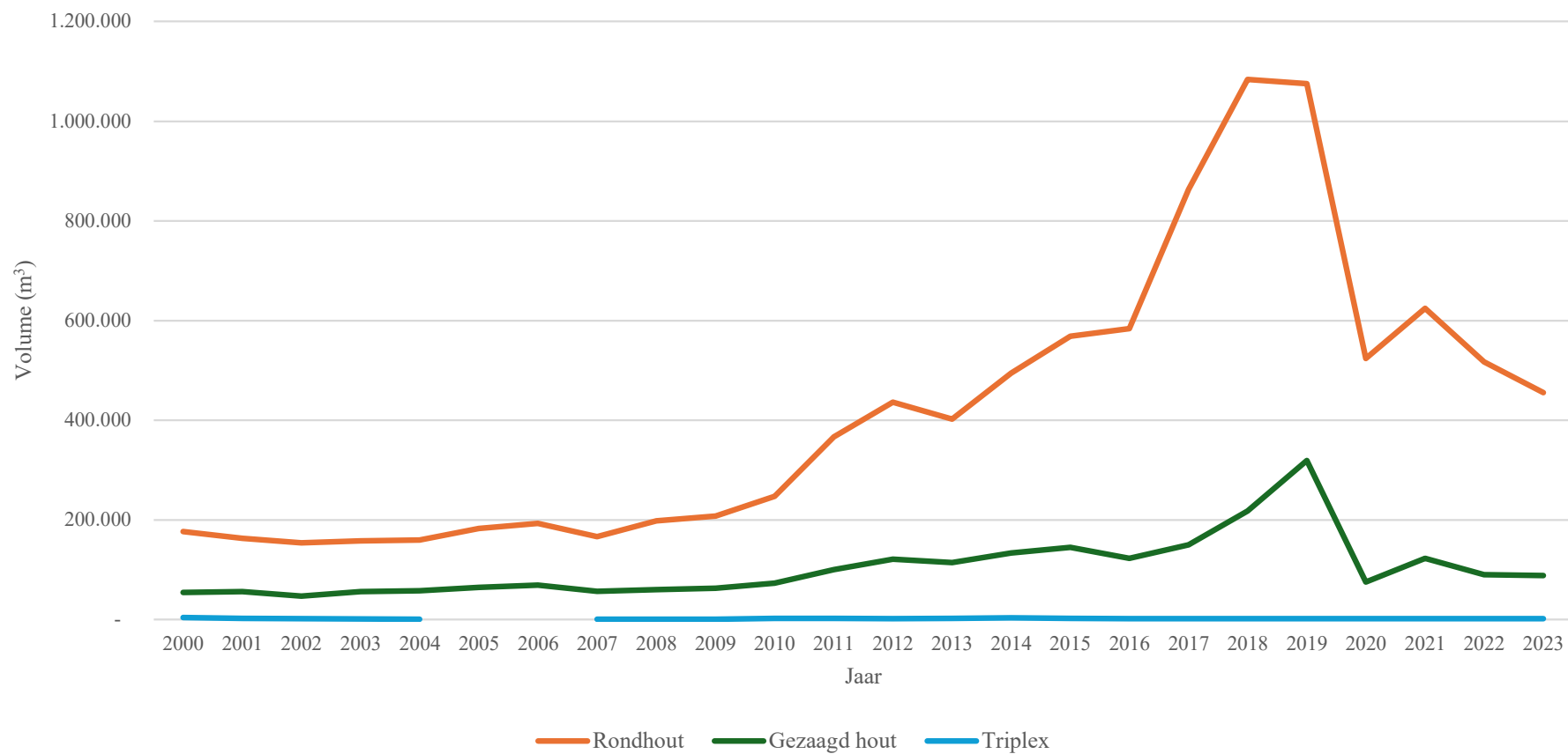
FIGUUR 3. HOUTPRODUCTIE 2000 - 2023
